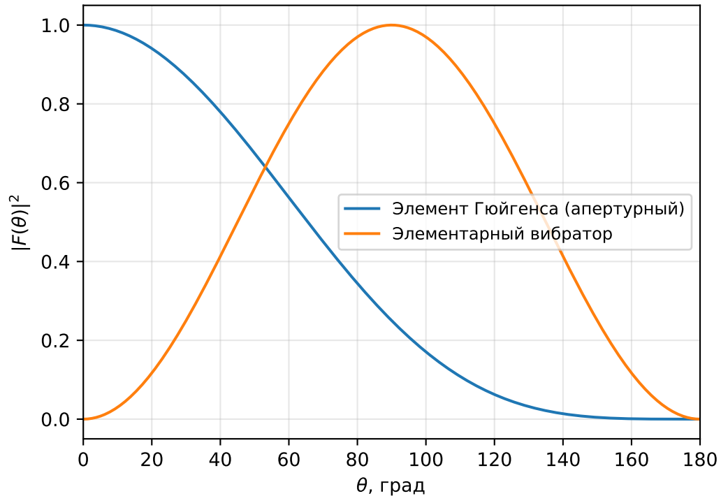
Нормированные ДН облучателей
