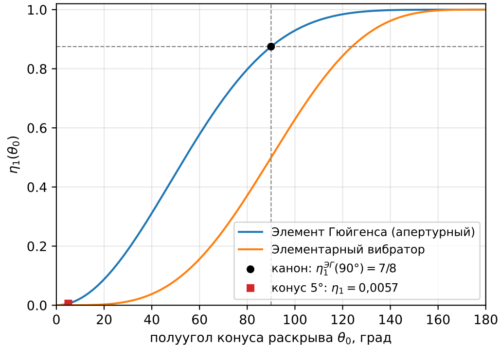
Перехват мощности раскрывом (spill-over)
